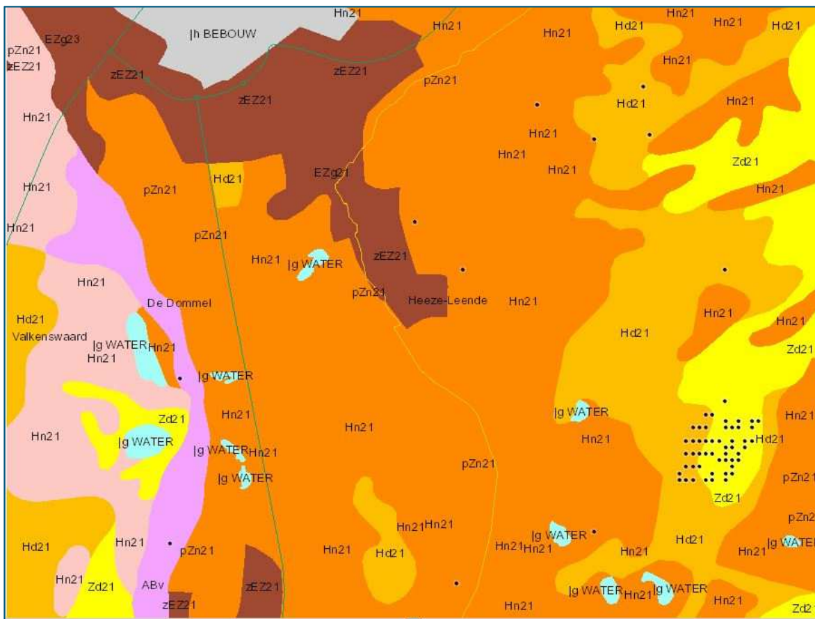
Figuur 4.2 Uitsnede Bodemkaart van Nederland zuidelijk deel projectgebied (bron: www.bodemdata.nl)
